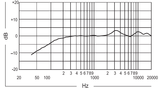
RESPUESTA DE FRECUENCIA TÍPICA FIGURA 1
