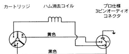
内部接続図
