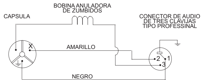
CONEXIONES INTERNAS FIGURA 2
