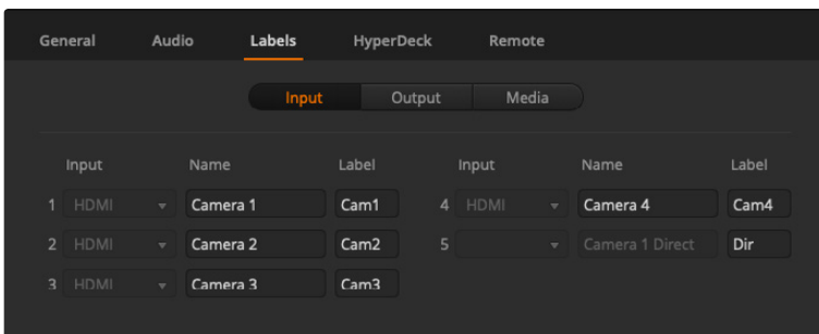
라벨 설정
