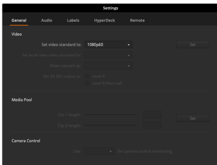
Finestra impostazioni
